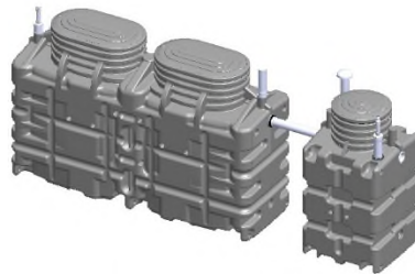
Vorklärung ST-1-5000 + Ecorock-1500, Ablaufklasse C
