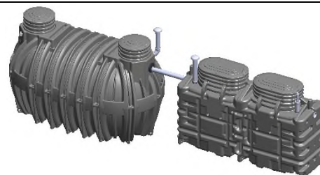
Vorklärung PT-1-10000 + Ecorock-5000, Ablaufklasse C
